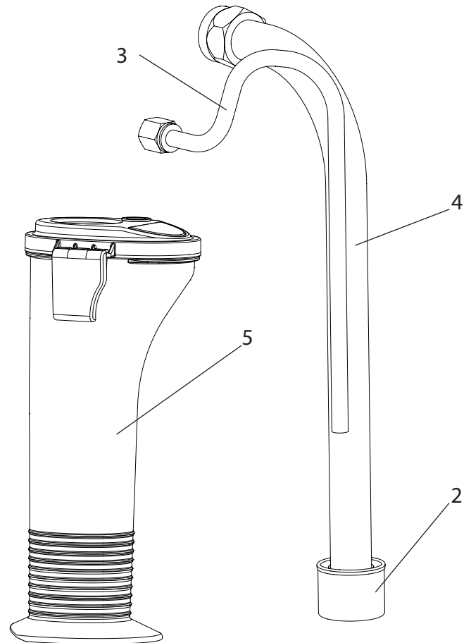
Onderdelenafbeelding aanzuigstelsysteem
