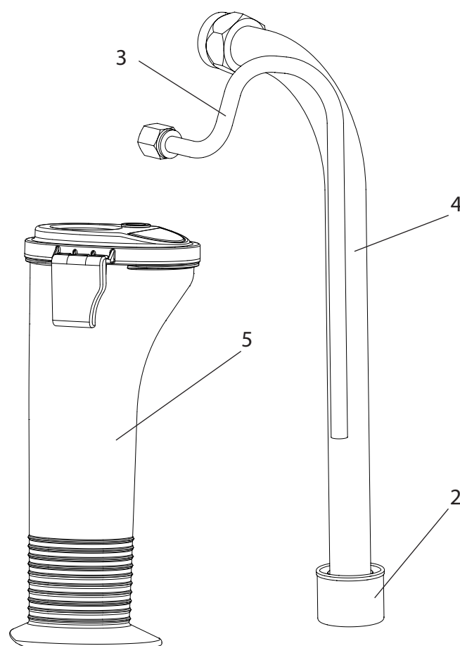
Reservedelsbillede, indsugningssystem
