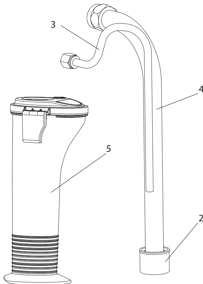
Reservdelsbild insugningssystem
