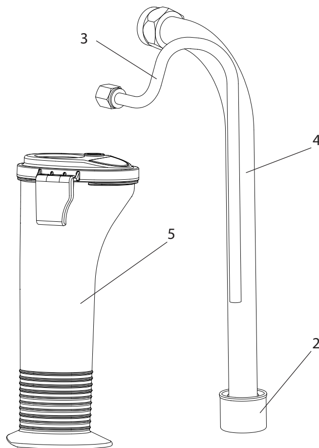
Reservedelsbillede, indsugningssystem
