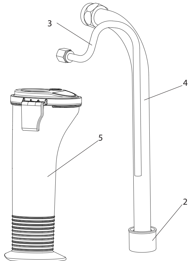
Cuadro de piezas de recambio sistema de aspiración
