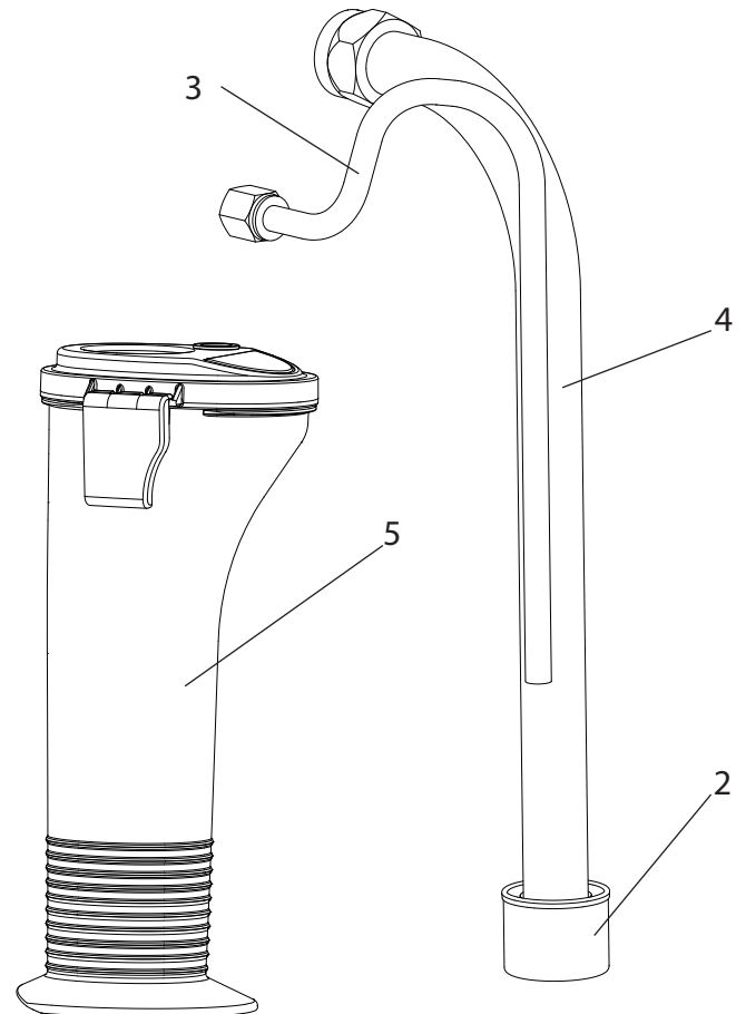
Onderdelenafbeelding aanzuigstelsysteem
