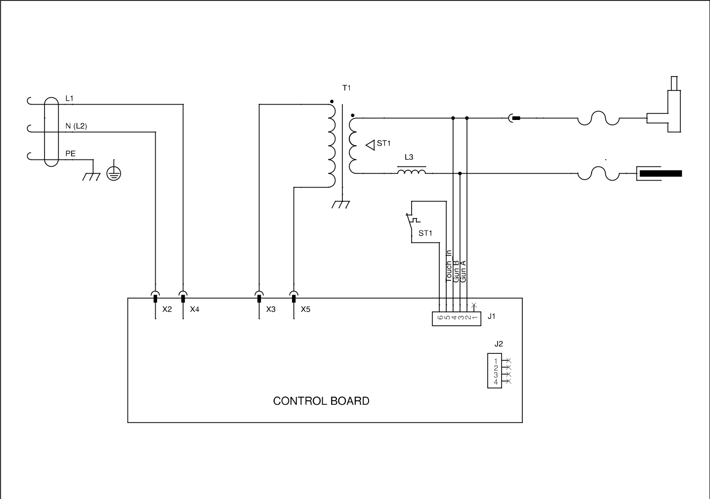
Schema elettrico, Schéma électrique, Diagram, Schaltplan, Esquema de conexiones.
