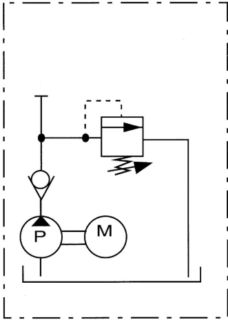
Esquema hidráulico Hydraulic circuit
