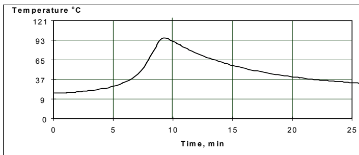
Curva típica exotérmica para el Plexus MA420, 23°C (10grams) 5
