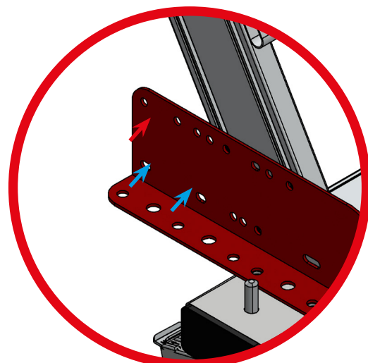
DETALLE 4
