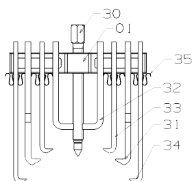
2 patas / 2 jaws
