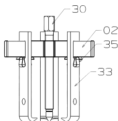
3 patas / 3 jaws
