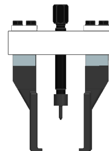
5075 Montado con alargador / 5075 assembled with the prolonger : A max 60 A min 20
